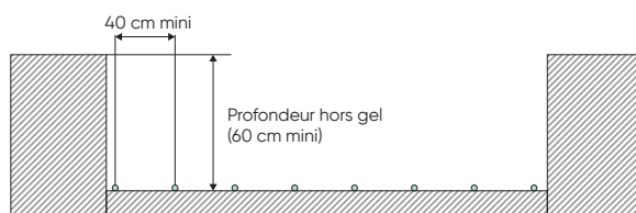
Pose après décapage (capteur sur une seule couche)
