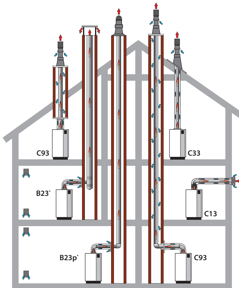
*Schéma de fumisterie avec conduit concentrique jusqu'au mur : obligatoire en hybrides gaz / non obligatoire en hybride fioul.
