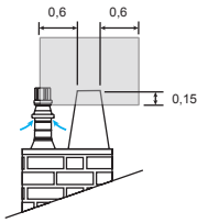
N Voisinage d'un conduit de fumée en tirage naturel
