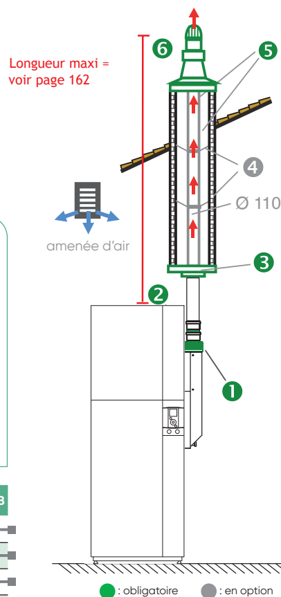
Conduit PPTL longueur 500 mm
