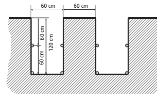
Pose en tranchées (capteur sur 2 couches)
