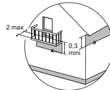
D Saillie de toiture ou de balcon (cas particuliers, voir NF DTU 61.1 P4)
