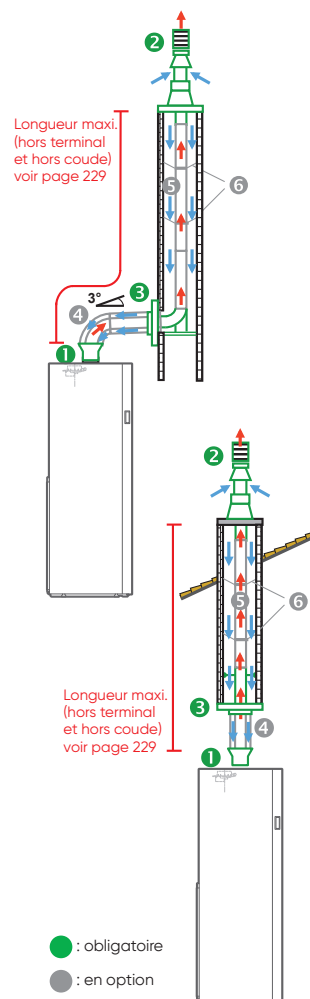
Raccord pour conduit flexible Ø80 à conduit flexible Ø80
